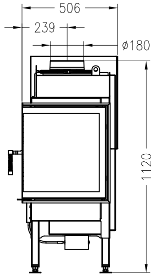
Seitenansicht M~1:20
